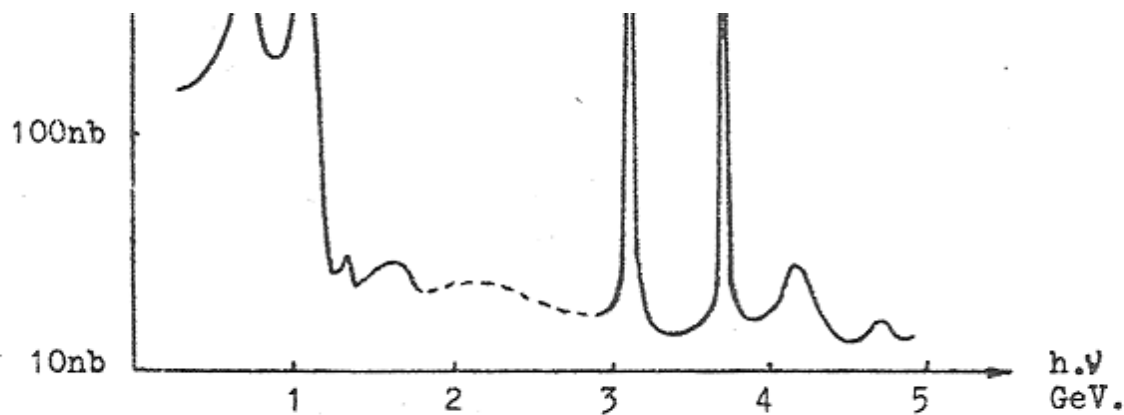
Fig. 1 - Courbes de résonance obtenues à STANFORD, dans l'étude des sections efficaces d'annihilation ( e^+, e^- ).
