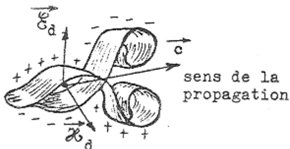
Fig. 2 - Configuration la plus probable des vortex disruptifs associés à un photon isolé.
